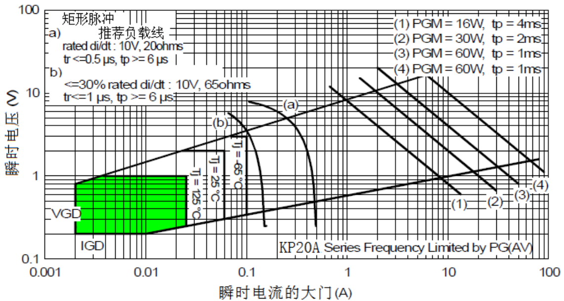
Fig. 16 - 栅极特性
